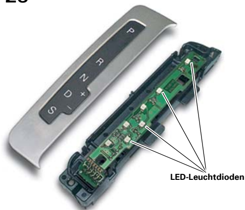
Anzeigeeinheit Y26
