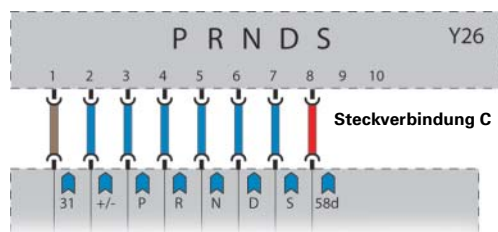
Wählhebelsensorik J587
