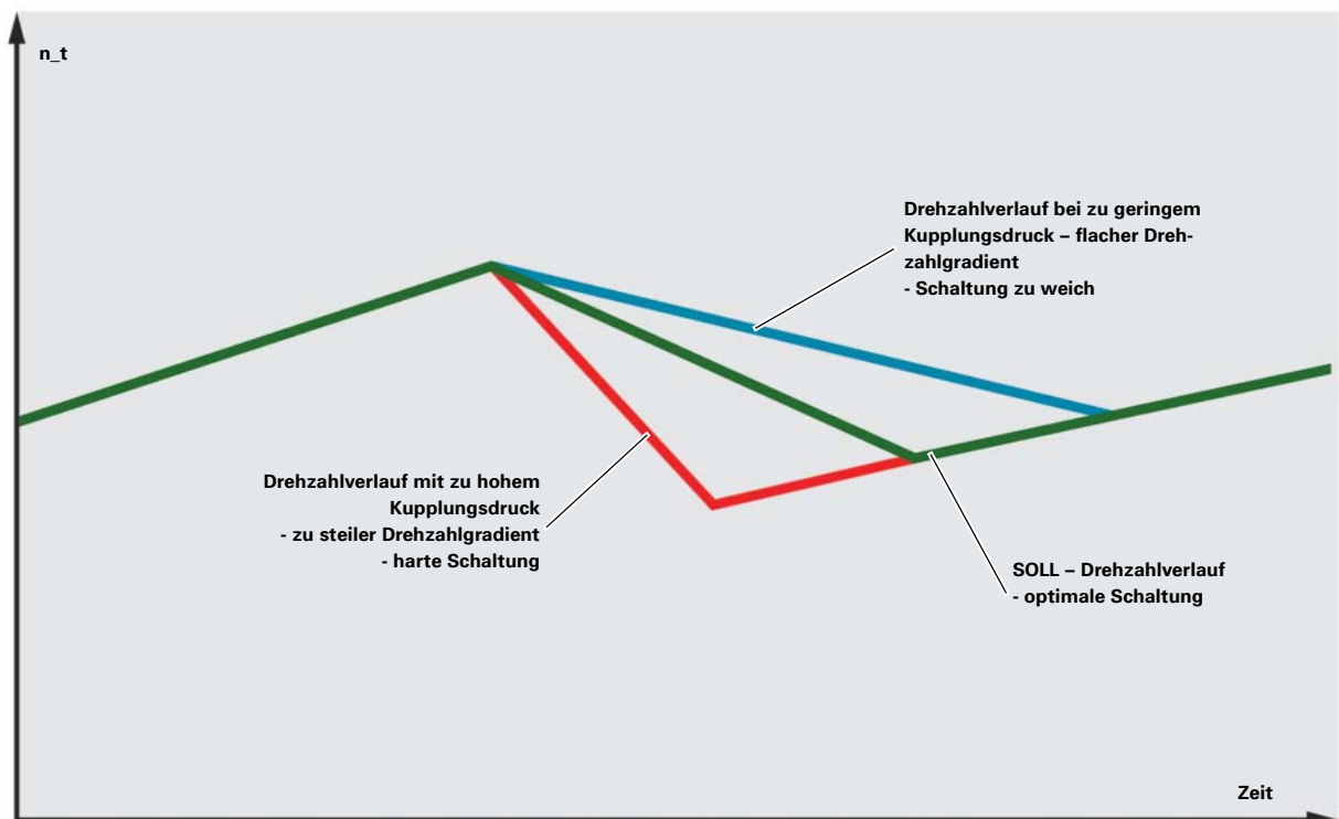
Exemplarische Darstellung des Drehzahlverlaufs bei einer Hochschaltung zur Veranschaulichung der Schaltadaption
