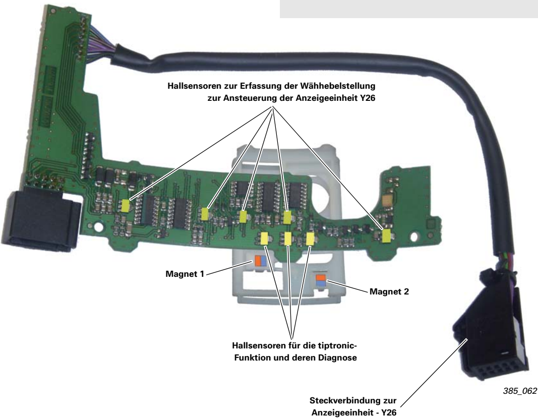
Wahlhebelsensorik J587
